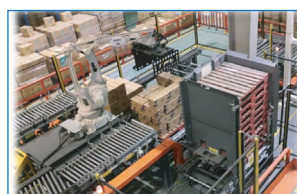
Máy xếp hàng lên Pallet Robot palletizing
