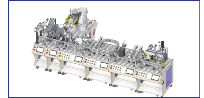
Hệ thống cơ điện tử MPS I4.0 MPS I4.0 mechatronic system
