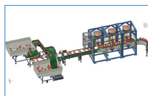
Hệ thống Robot cấp chai Robotic bottle unscrambler
