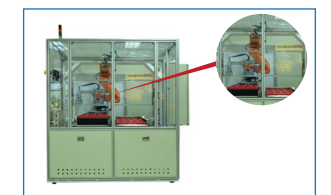
Máy cấp màn hình cảm ứng sử dụng robot 6 trục The touch screen feeder uses a 6-axis robot
