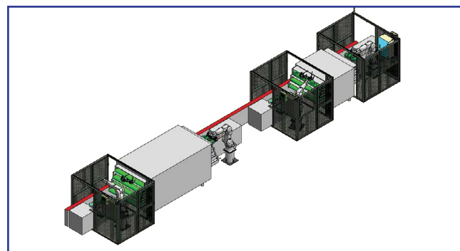
Dây chuyền robot gấp sản phẩm Công ty TNHH điện tử Foster Pick & place robot - Foster
