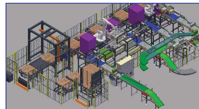
Hệ thống Palletizer 4 in 4 out Nhà máy Unilever Củ Chi Robot Palletizer 4 in 4 out system - Unilever Cu Chi
